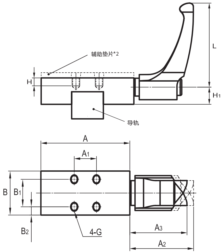
尺寸图
