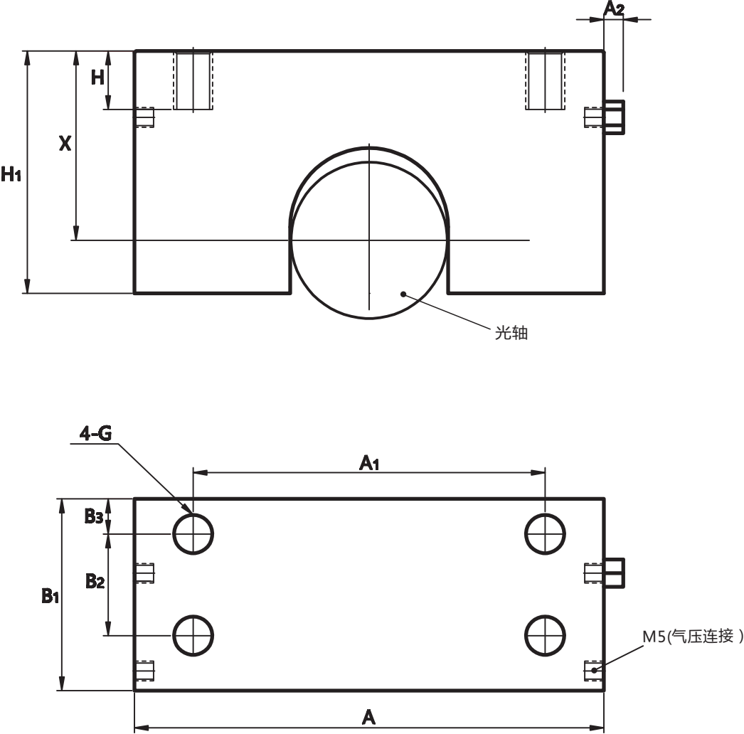
尺寸图
