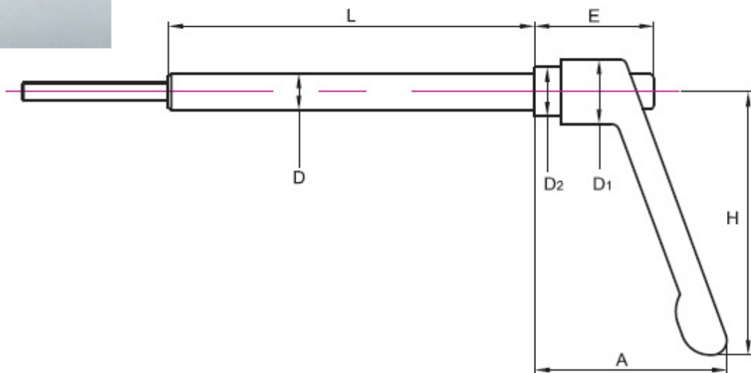
尺寸图
