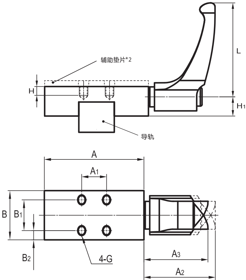
尺寸图
